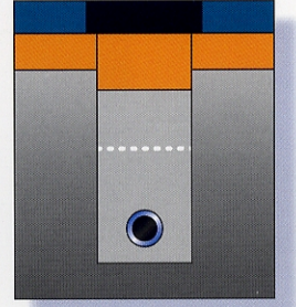
Yerleştirme yatağı, kaplama, doldurma
